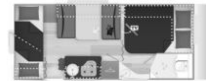
EVOLUTION 510PE KIDS • 5,20 x 2,15 m
